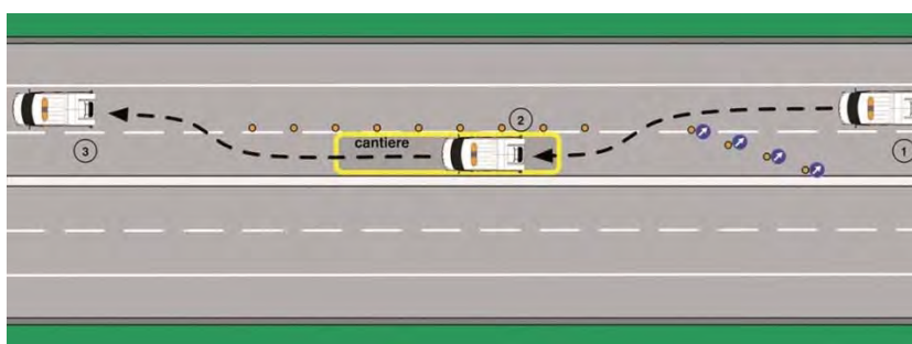
Figura 7 – Manovra di accesso e uscita dai cantieri in caso di chiusura della corsia di sorpasso
