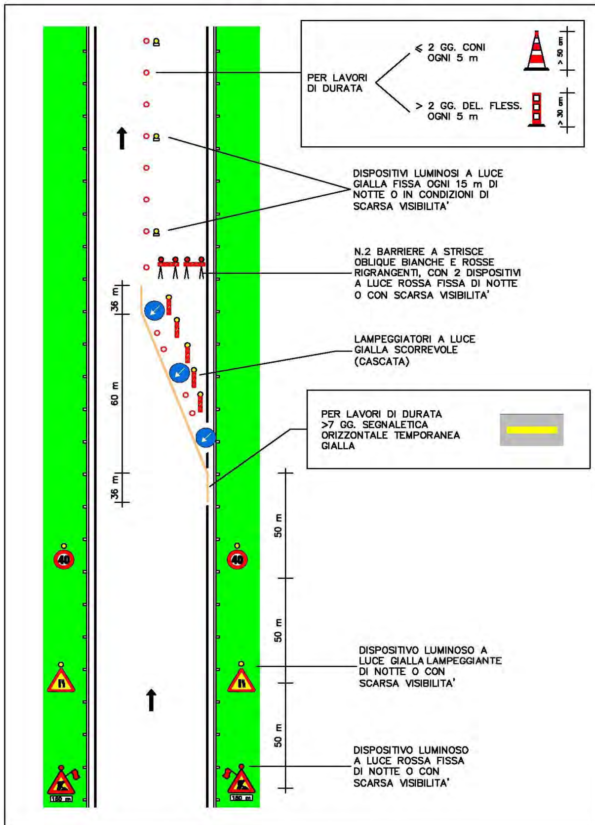
CHIUSURA DI UNA SEMICARREGGIATA SU RAMI DI SVINCOLO A SENSO UNICO
