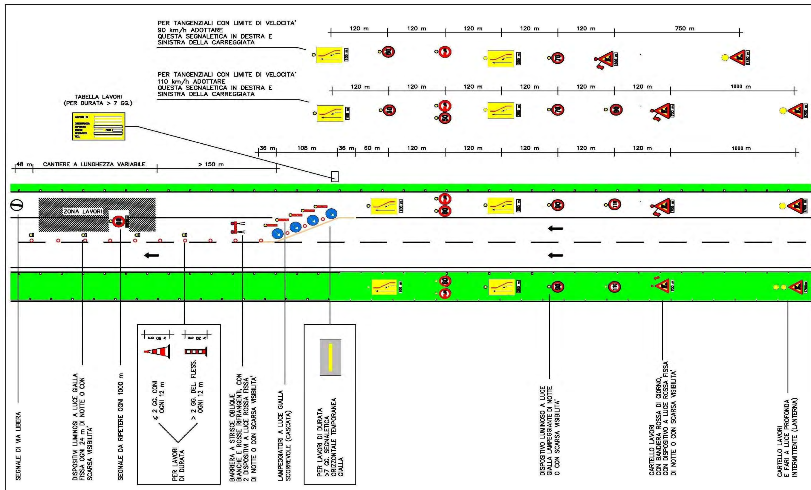
CHIUSURA DELLA CORSIA DI MARCIA IN AUTOSTRADA CON 2 CORSIE
