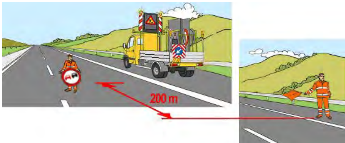
Figura 22 – Chiusura della corsia di marcia: installazione della segnaletica
