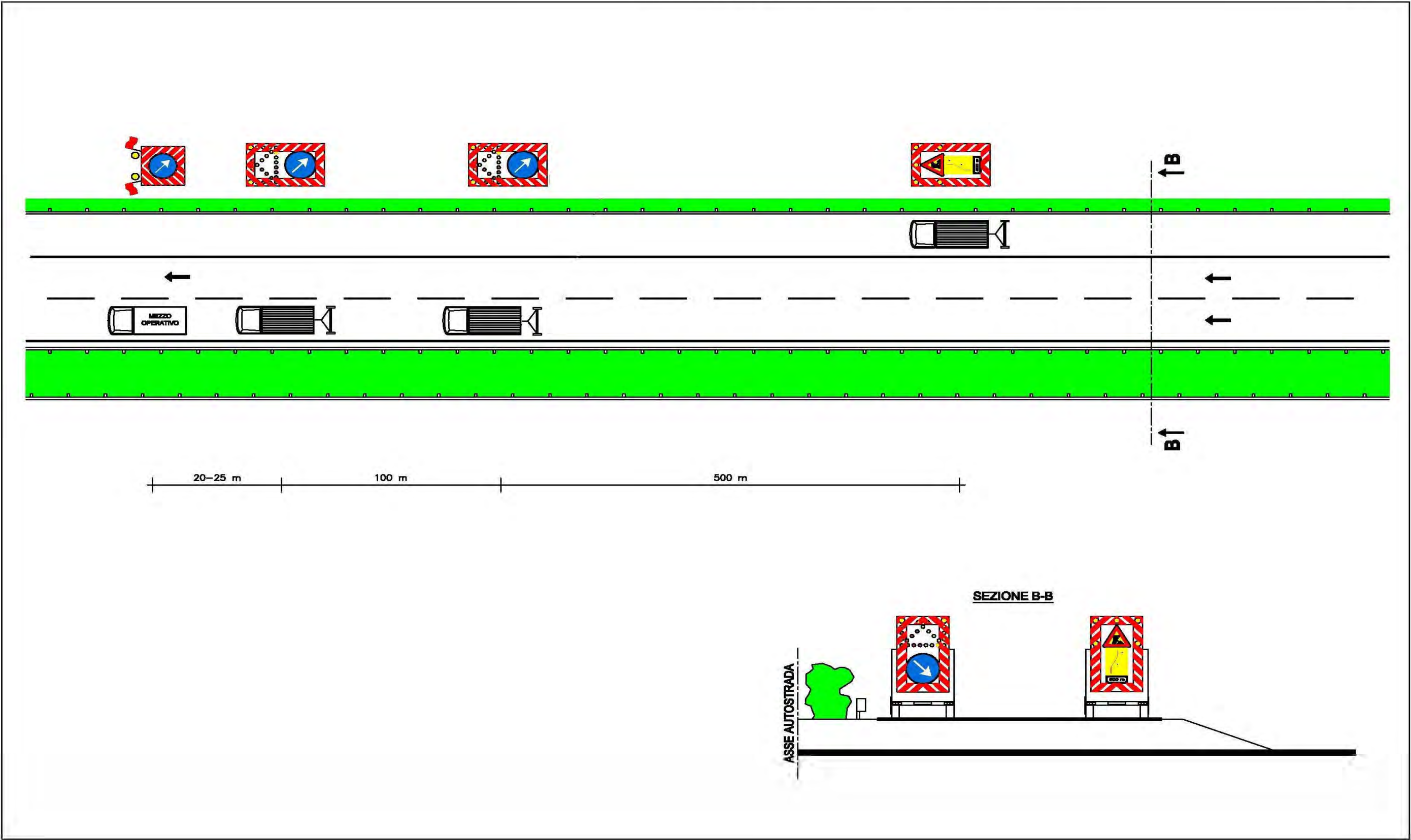
CANTIERE MOBILE CON CHIUSURA DELLA CORSIA DI SORPASSO, PER LAVORI, CONTROLLI, SONDAGGI E VERIFICHE DI RAPIDA ESECUZIONE IN AUTOSTRADA CON 2 CORSIE O TANGENZIALI CON CORSIA DI EMERGENZA
